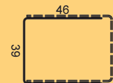
2) 12 \varnothing 8 L=131cm
