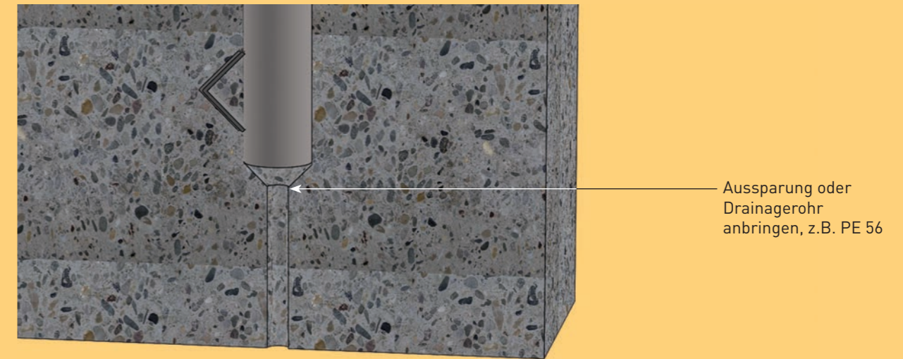
Sickerlage Rundkies 16-32
